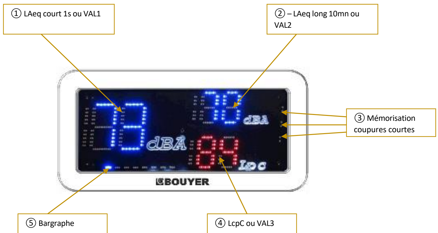
Figure 3. L'afficheur AF-VAL1 – Vue de face
