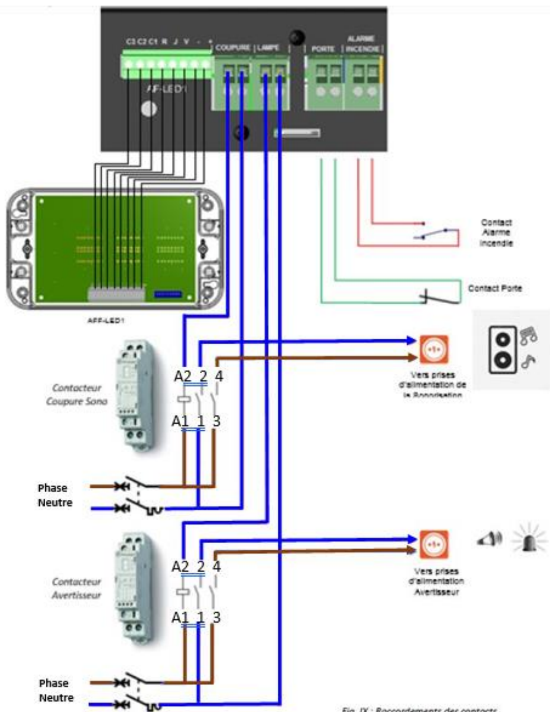
Fig. IX : Raccordements des contacts
