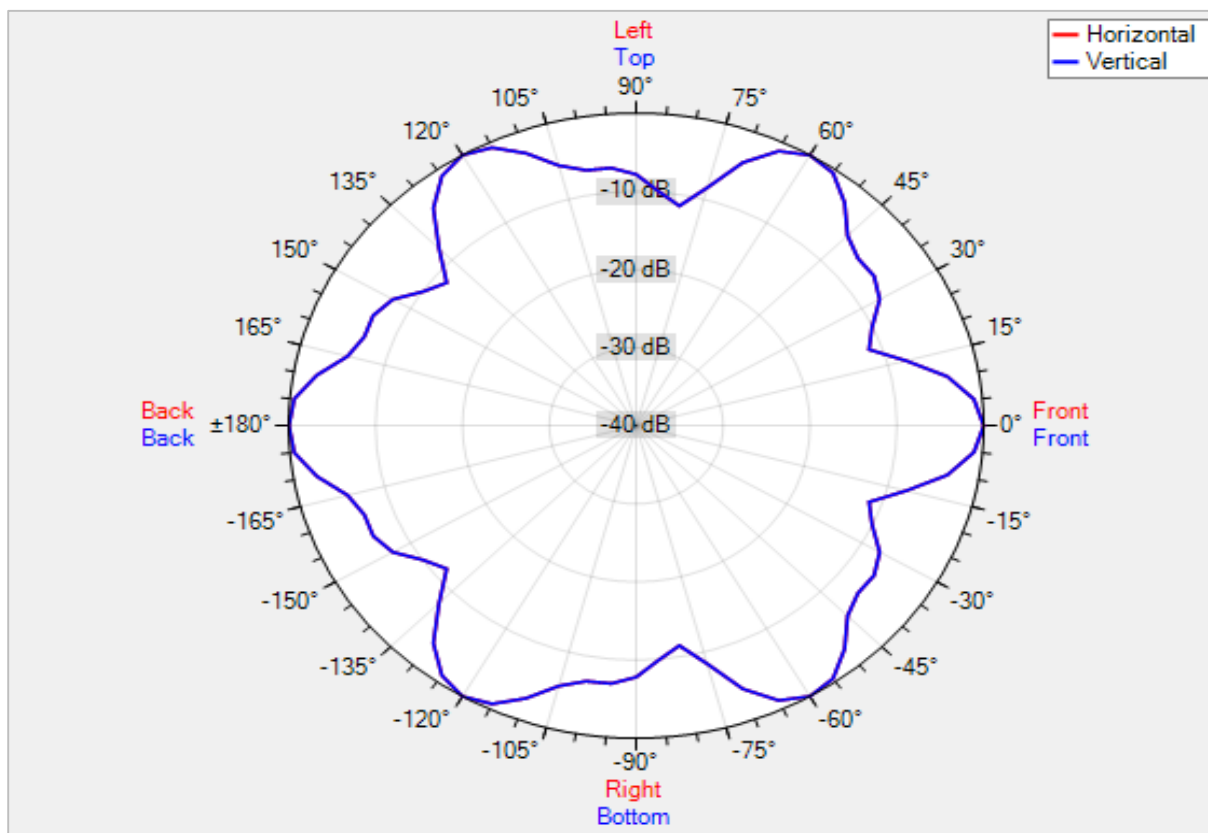
Directivité à 1 KHz
