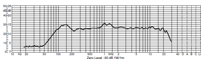
Courbe de réponse / Frequency response
